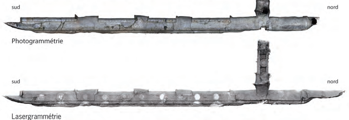
Figure 34 Comparaison des nuages denses, en haut la photogrammétrie et en bas la lasergrammétrie. © V. Mialhe (SahCM)
