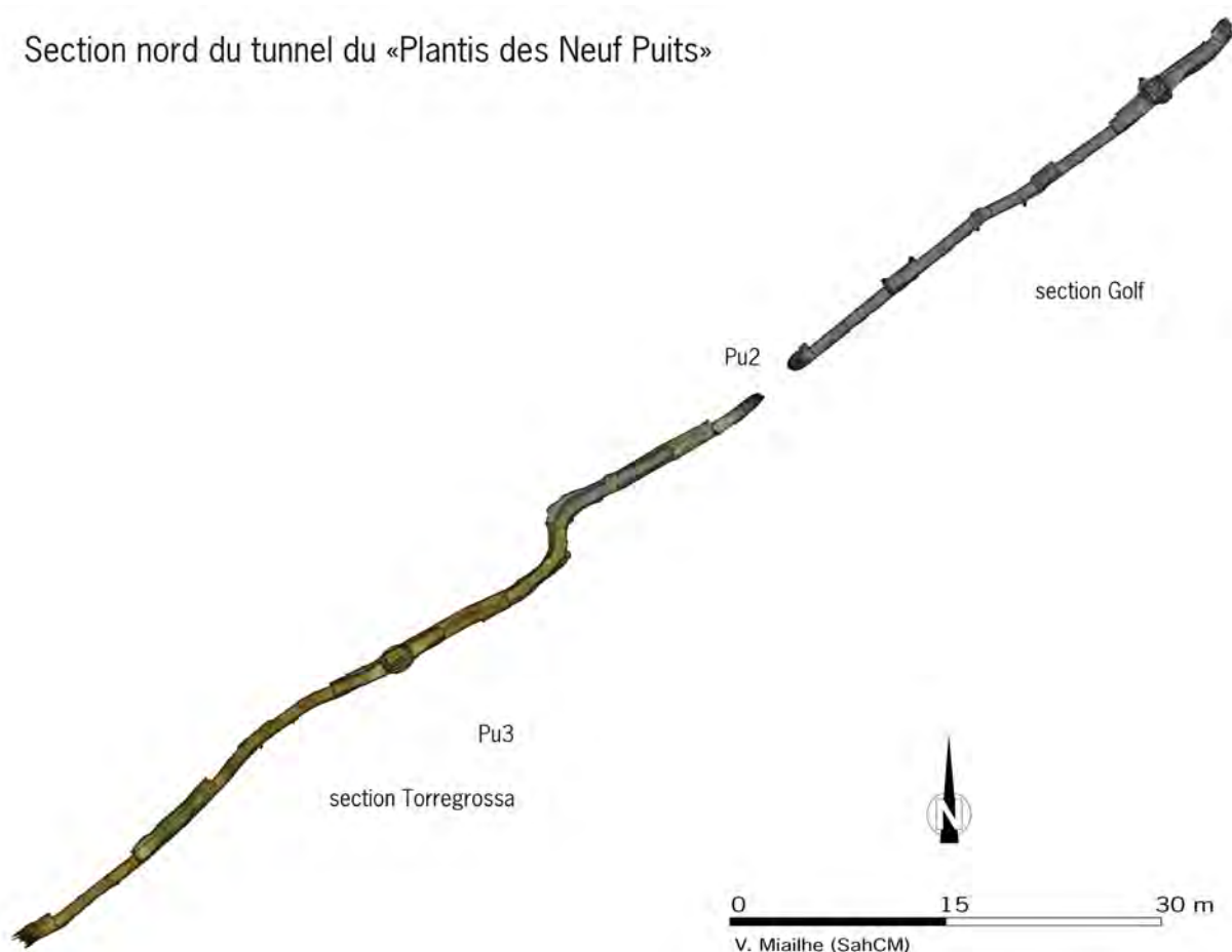
Figure 61 Les inflexions du tracé de la section nord du tunnel du « Plantis des Neuf Puits » issu de la photogrammétrie. © V. Miaillhe (SahCM)
