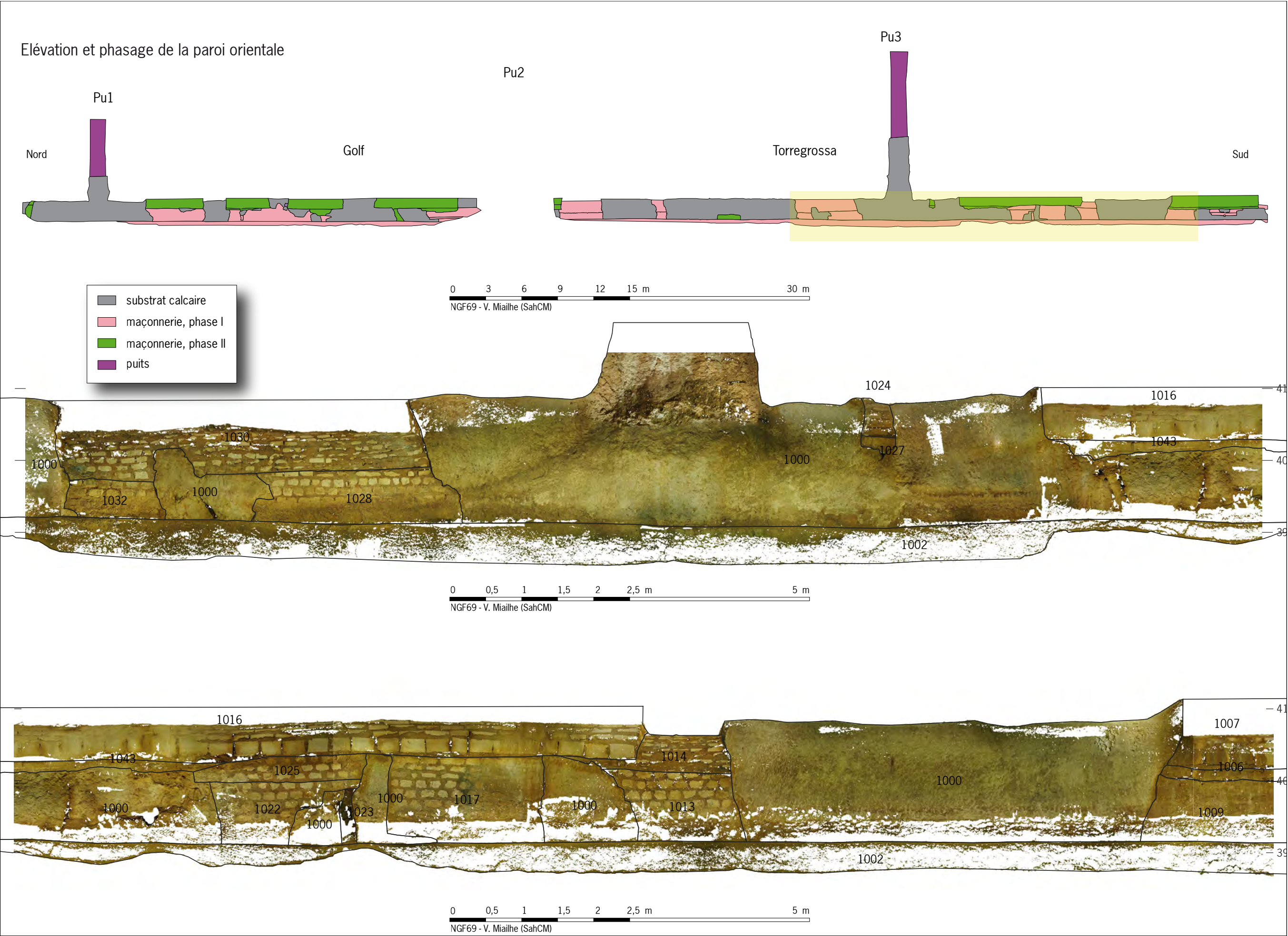
Figure 70 Élévation par nuage dense et phasage de la paroi orientale des sections souterraines du Golf et de Torregrossa, zone 3. © V. Mialhe (SahCM)
