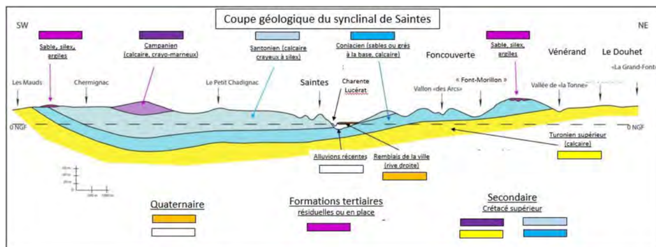
Figure 11 Coupe géologique de Saintes.
