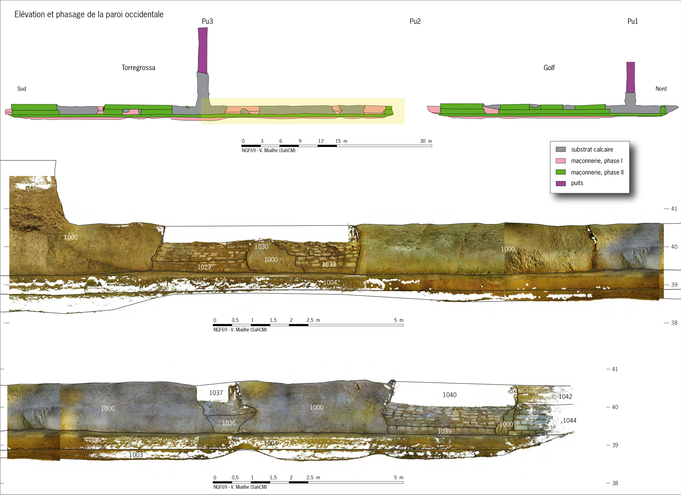
Figure 65 Élévation par nuage dense et phasage de la paroi occidentale des sections souterraines du Golf et de Torregrossa, zone 2. © V. Mialhe (SahCM)
