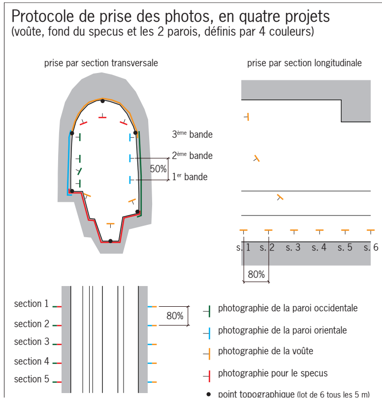
Figure 29 Protocole de prise de photos dans le tunnel pour les levés photogrammétriques. © V. Mialhe (SahCM)
