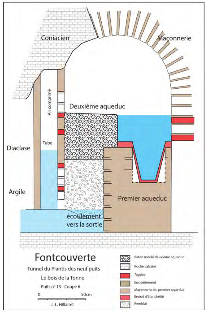
Figure 81 Coupe du conduit dans la section du « Bois de la tonne ». © J.-L. Hillairet (SahCM)
