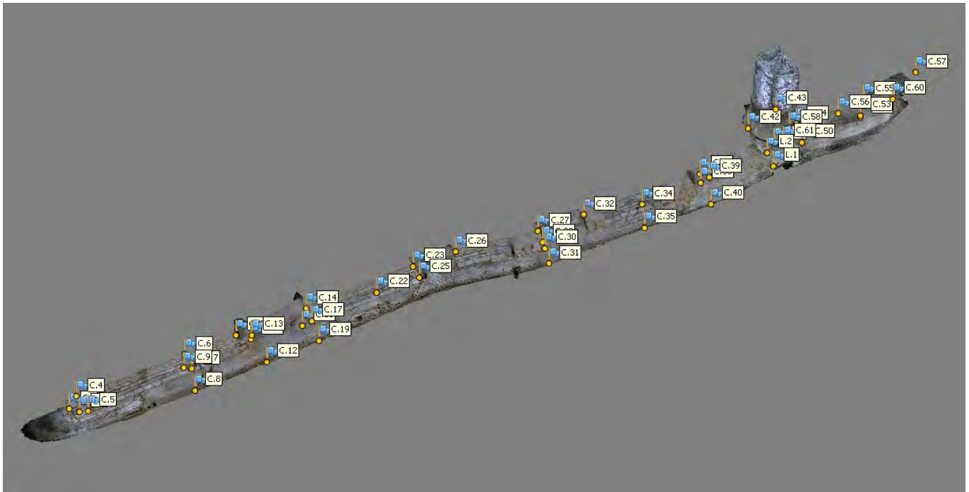
Figure 30 Répartition des cibles géodésiques pour la photogrammétrie, à l'intérieur du conduit du Golf. © V. Mialhe (SahCM)
